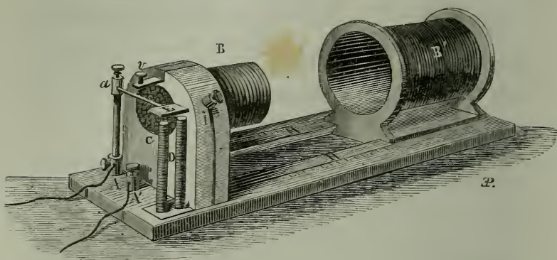
FIG. 71. — Appareil volta-faradique de Du Bois-Reymond.
